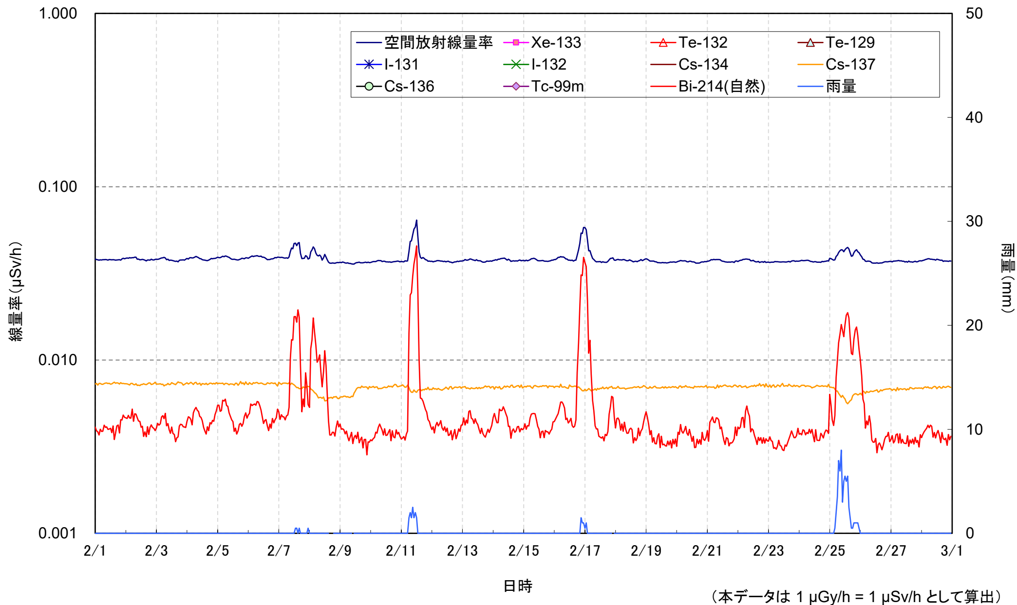
日本分析センターにおける空間放射線量率の測定結果(2026年2月)
