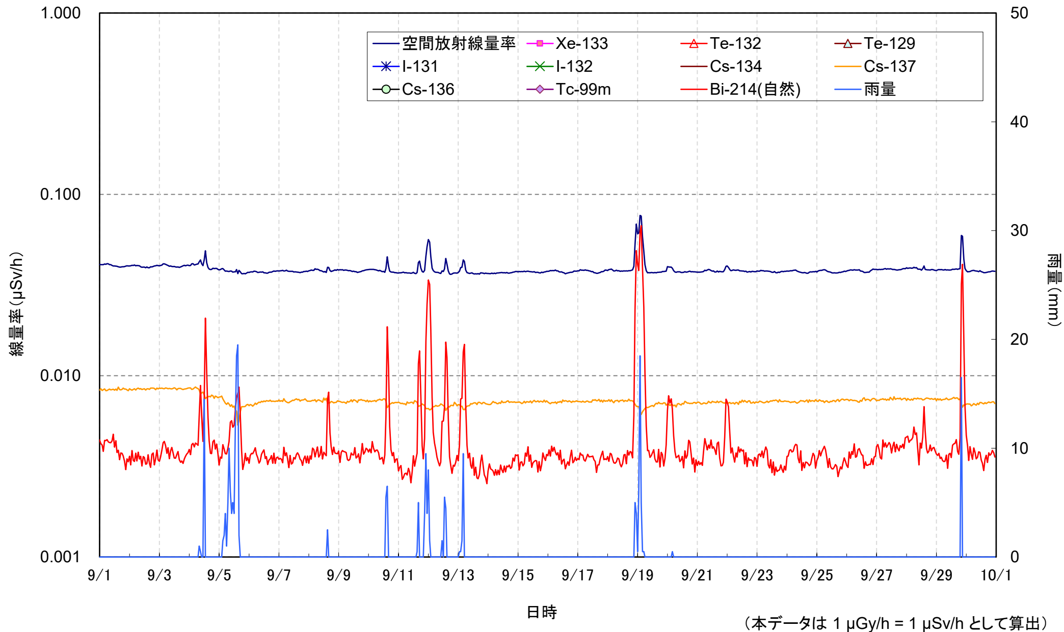
日本分析センターにおける空間放射線量率の測定結果(2025年9月)
