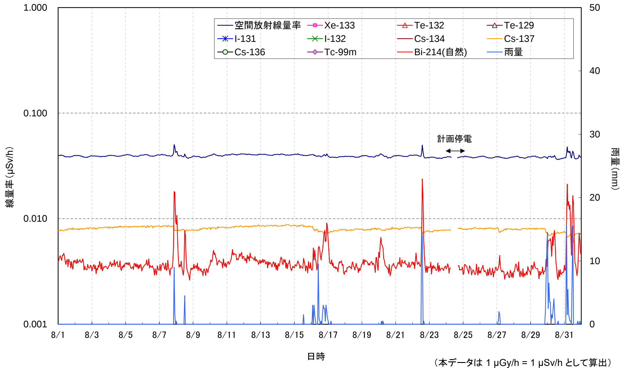
日本分析センターにおける空間放射線量率の測定結果(2024年 8月)
