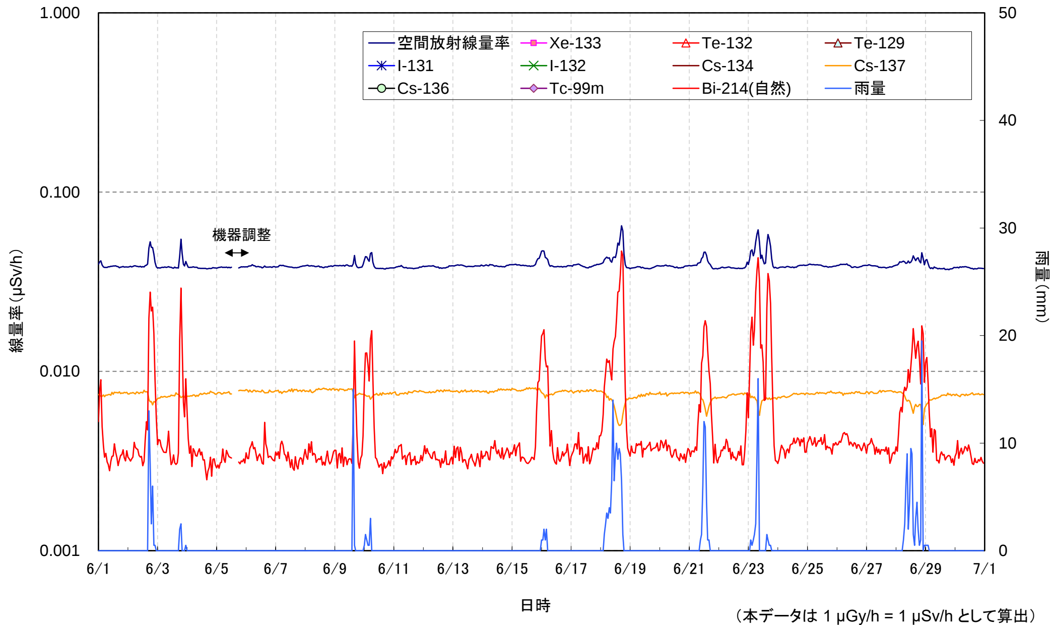
日本分析センターにおける空間放射線量率の測定結果(2024年6月)
