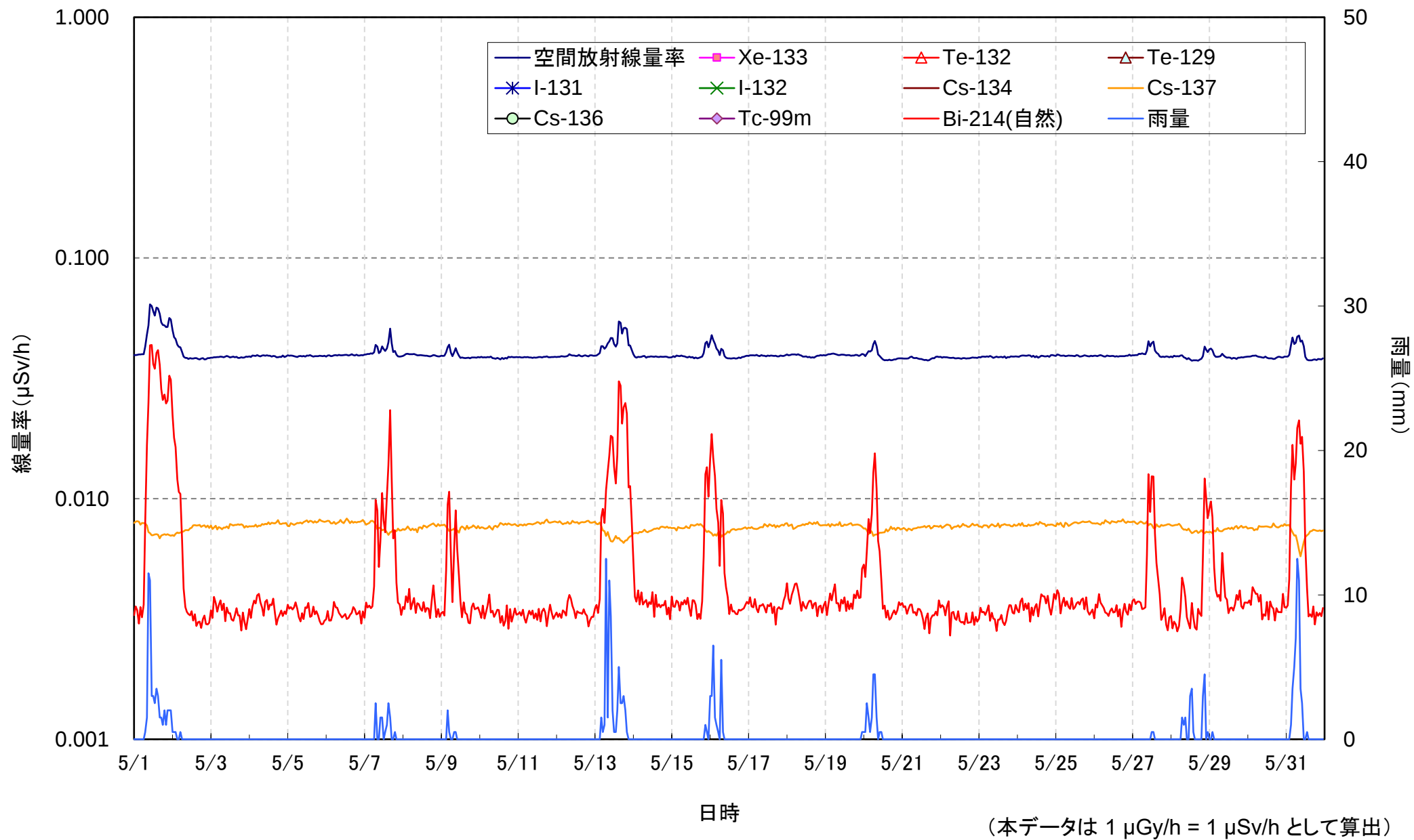
日本分析センターにおける空間放射線量率の測定結果(2024年 5月)
