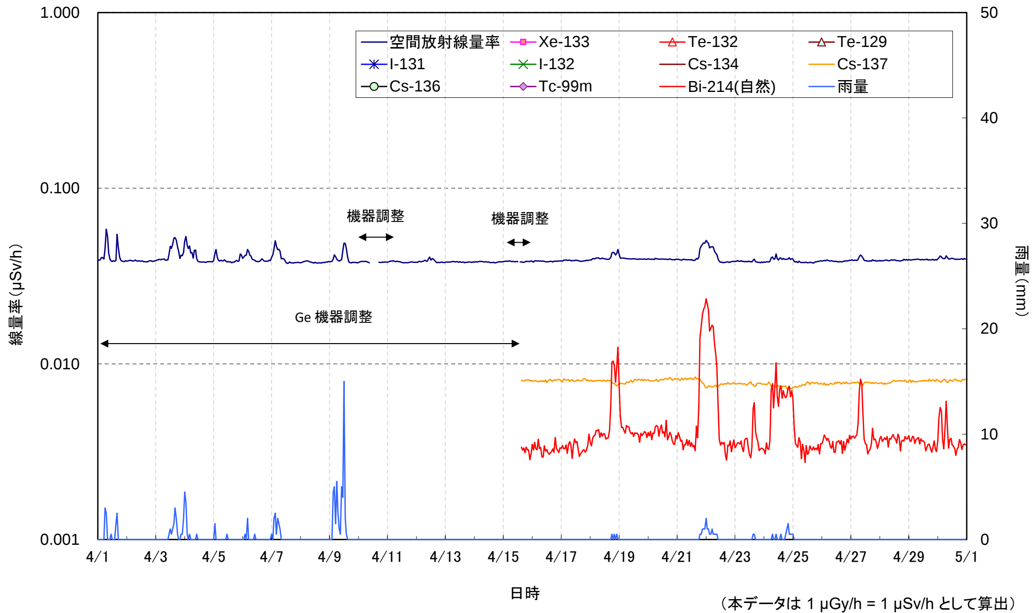
日本分析センターにおける空間放射線量率の測定結果(2024年 4月)
