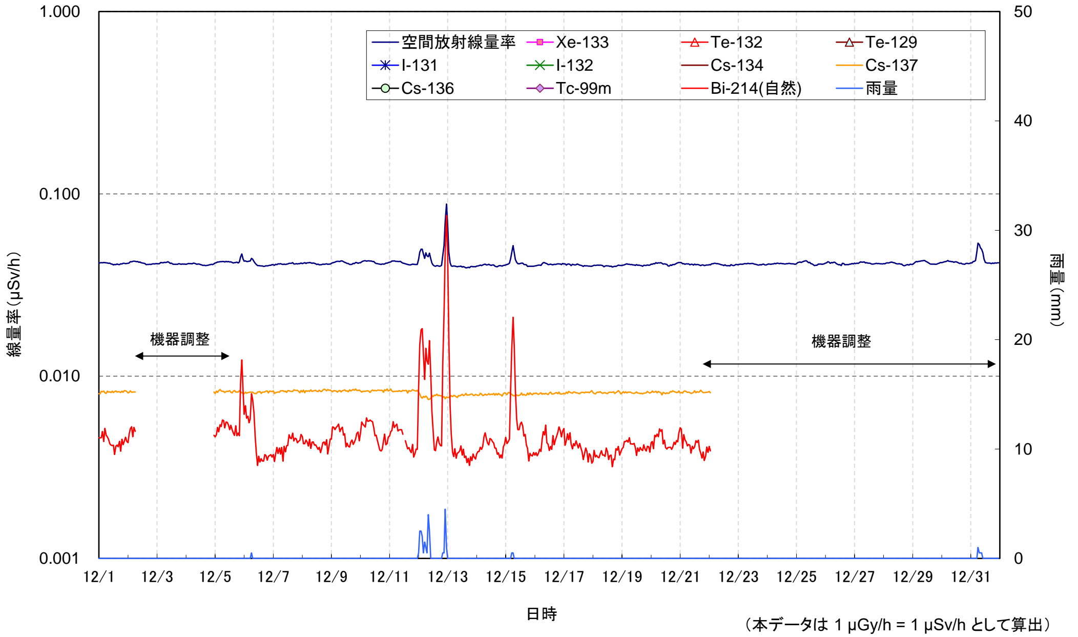
日本分析センターにおける空間放射線量率の測定結果(2023年12月)
