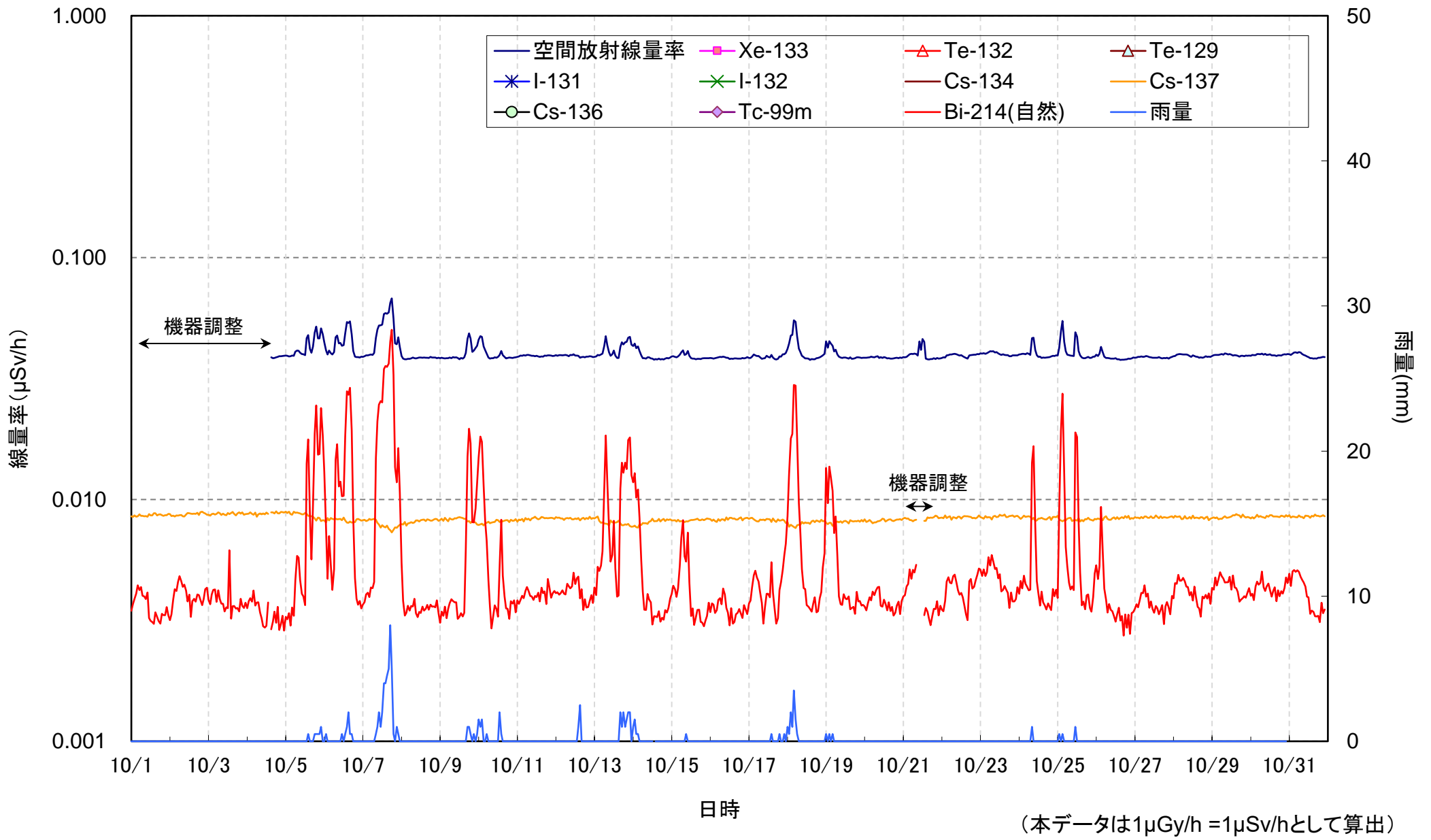
日本分析センターにおける空間放射線量率の測定結果(2022年10月)
