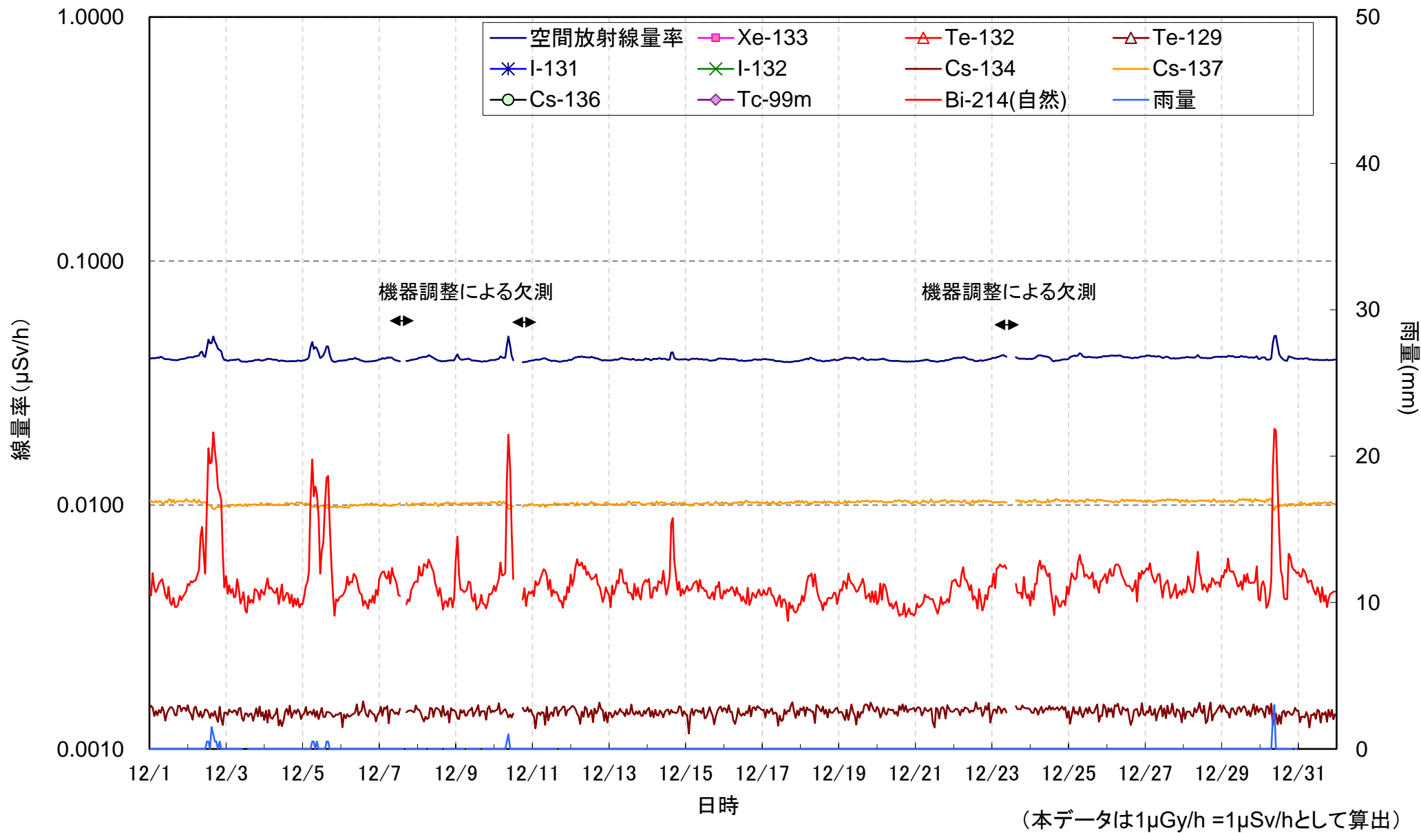
日本分析センターにおける空間放射線量率の測定結果(2020年12月)
