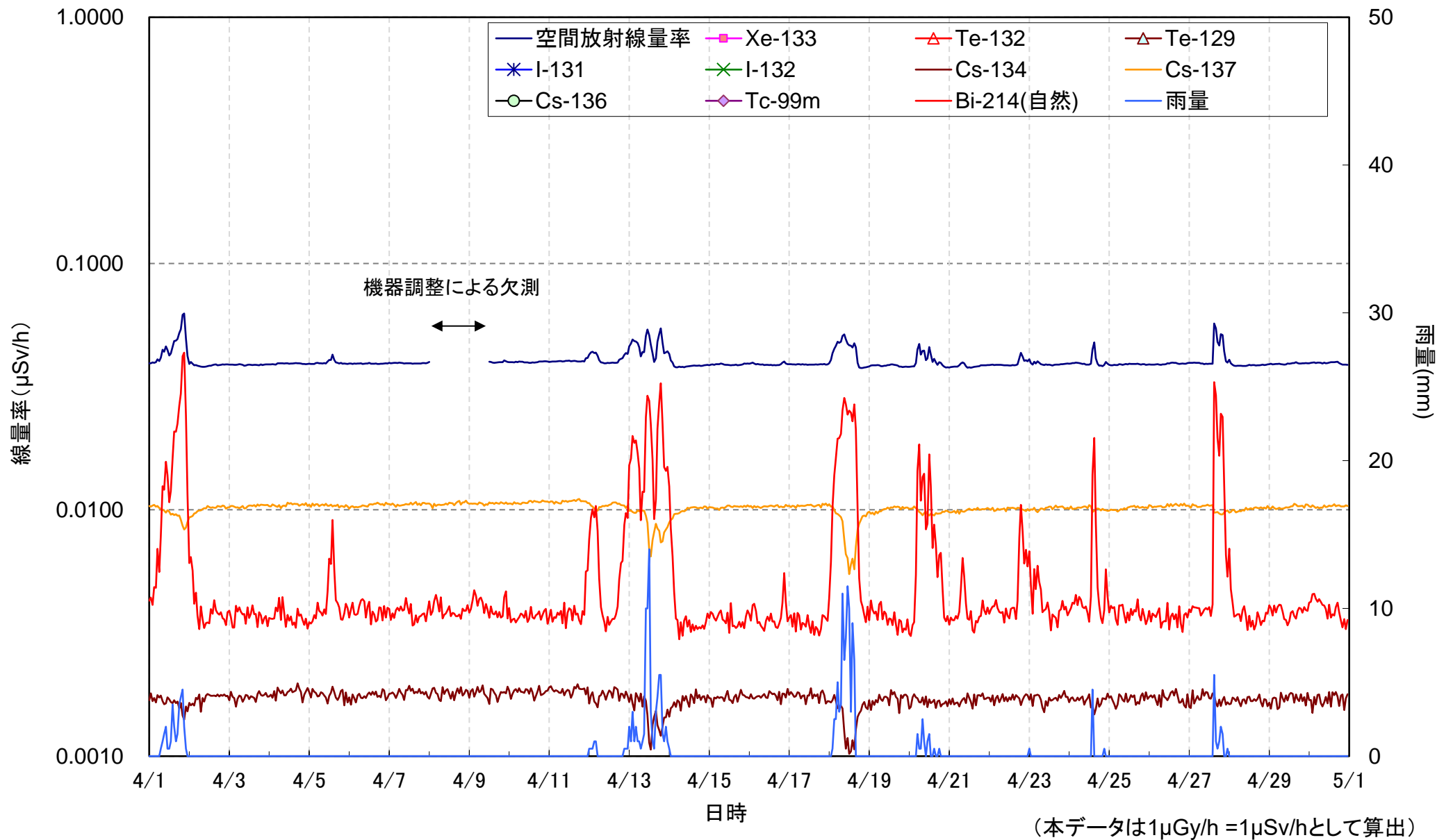
日本分析センターにおける空間放射線量率の測定結果(2020年4月)
