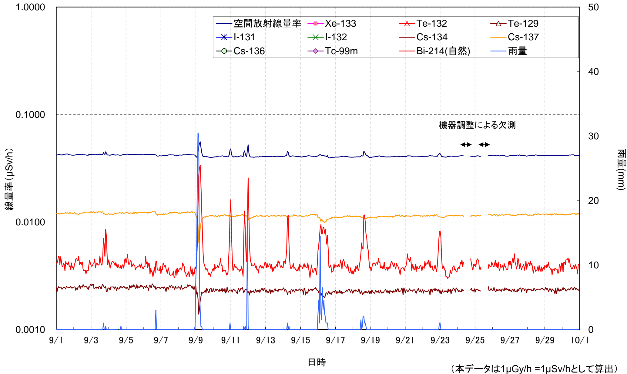
日本分析センターにおける空間放射線量率の測定結果(2019年9月)
