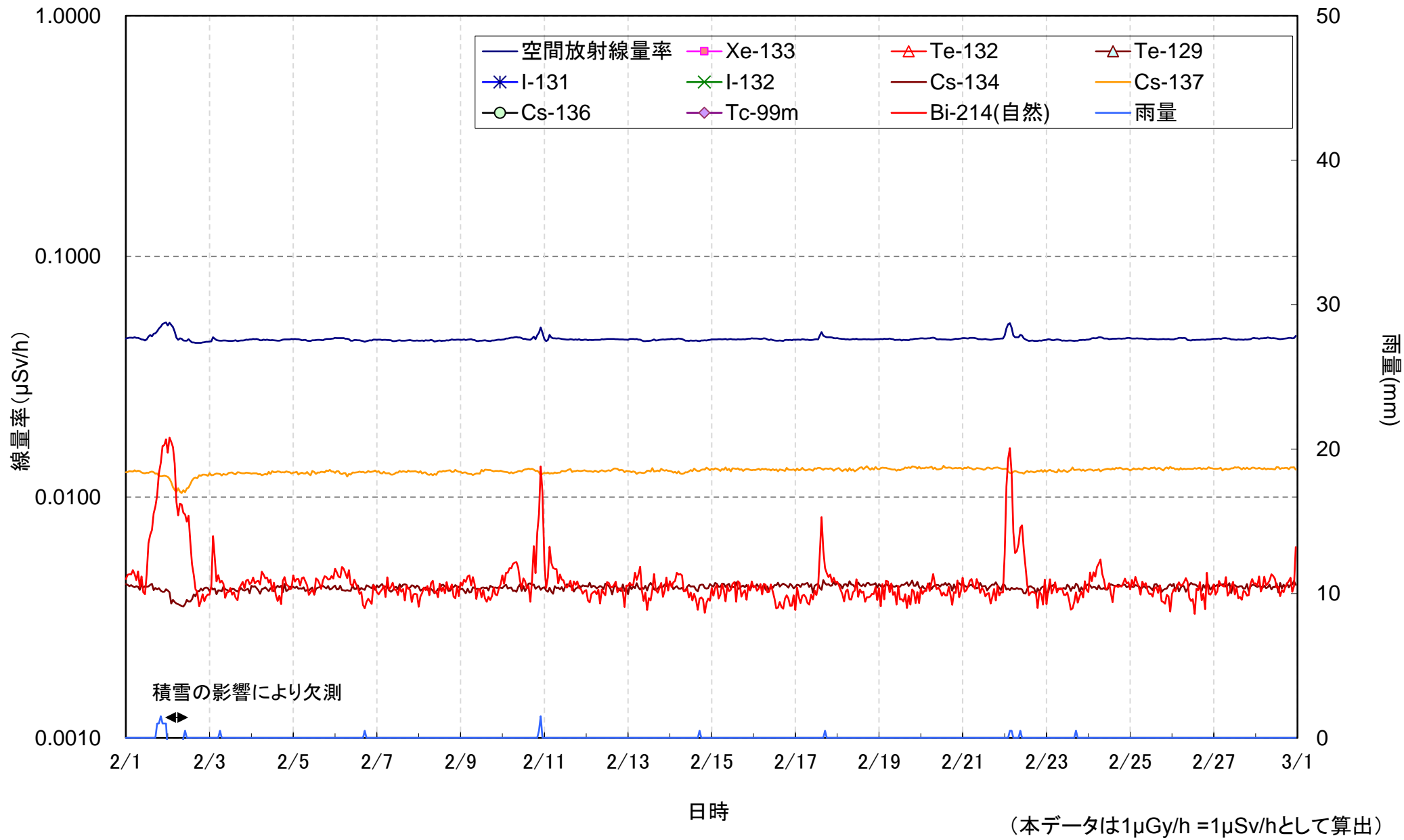
日本分析センターにおける空間放射線量率の測定結果(2018年2月)
