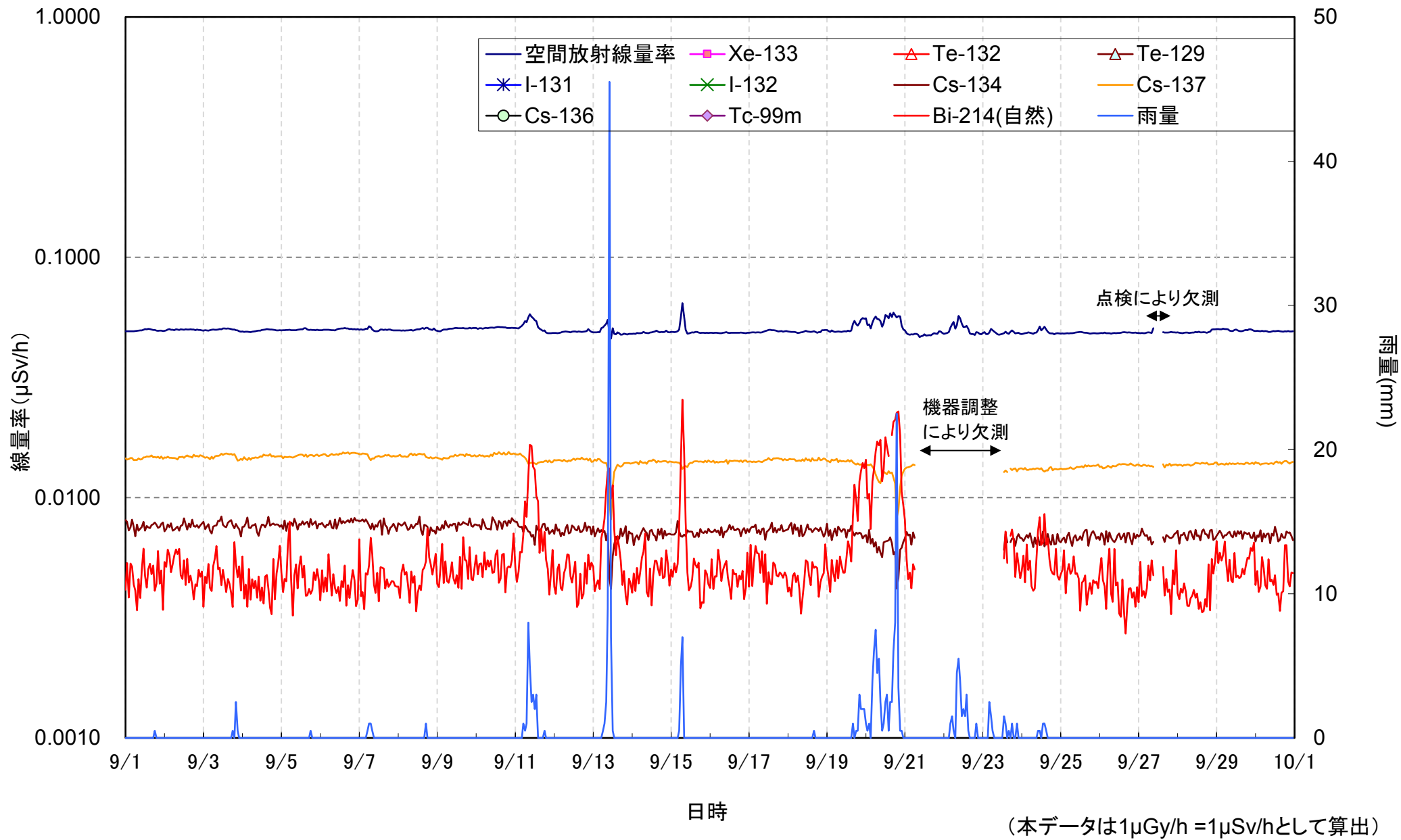
日本分析センターにおける空間放射線量率の測定結果(2016年9月)
