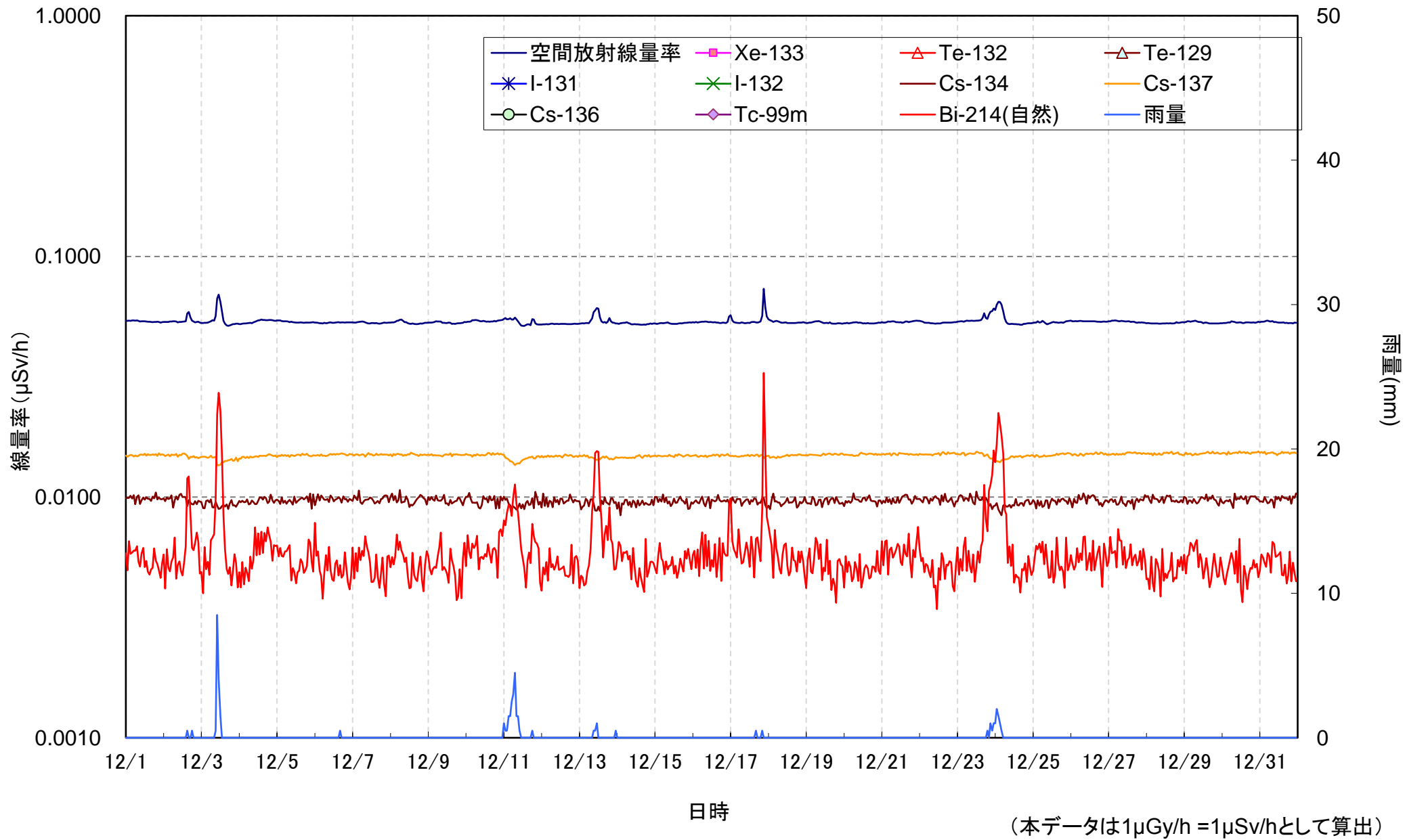
日本分析センターにおける空間放射線量率の測定結果(2015年12月)
