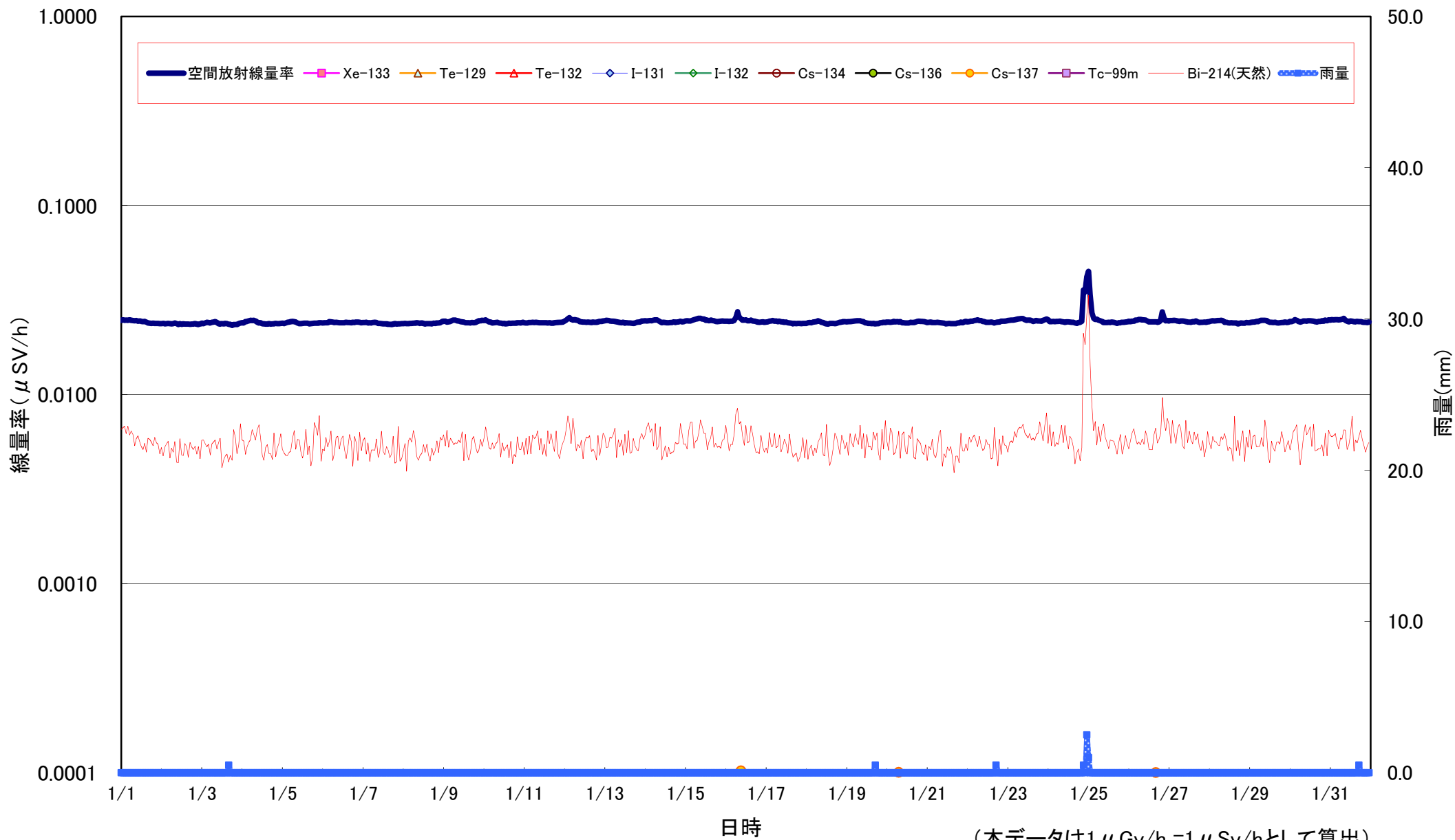
日本分析センターにおける空間放射線量率の測定結果(2011年1月:事故前)
