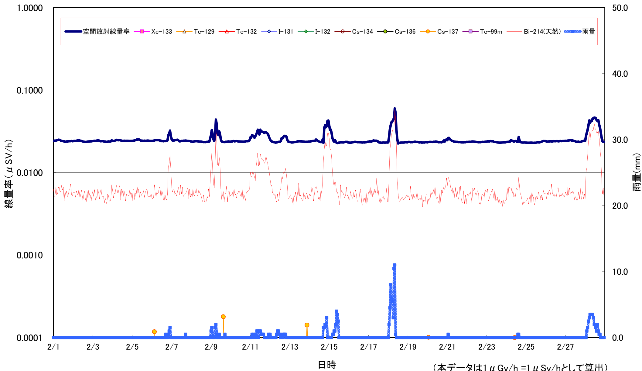
日本分析センターにおける空間放射線量率の測定結果(2011年2月:事故前)
