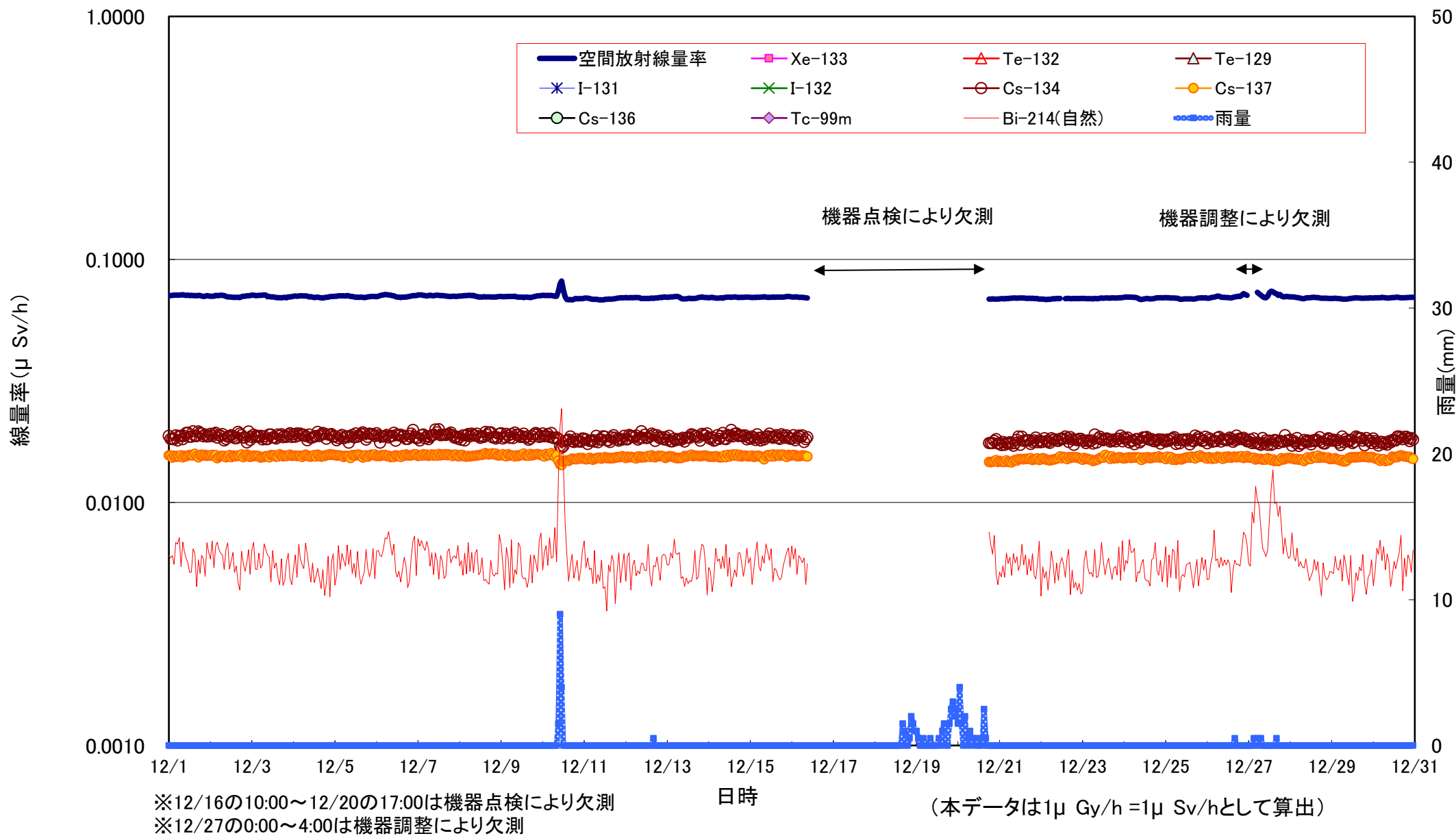
日本分析センターにおける空間放射線量率の測定結果(2013年12月)
