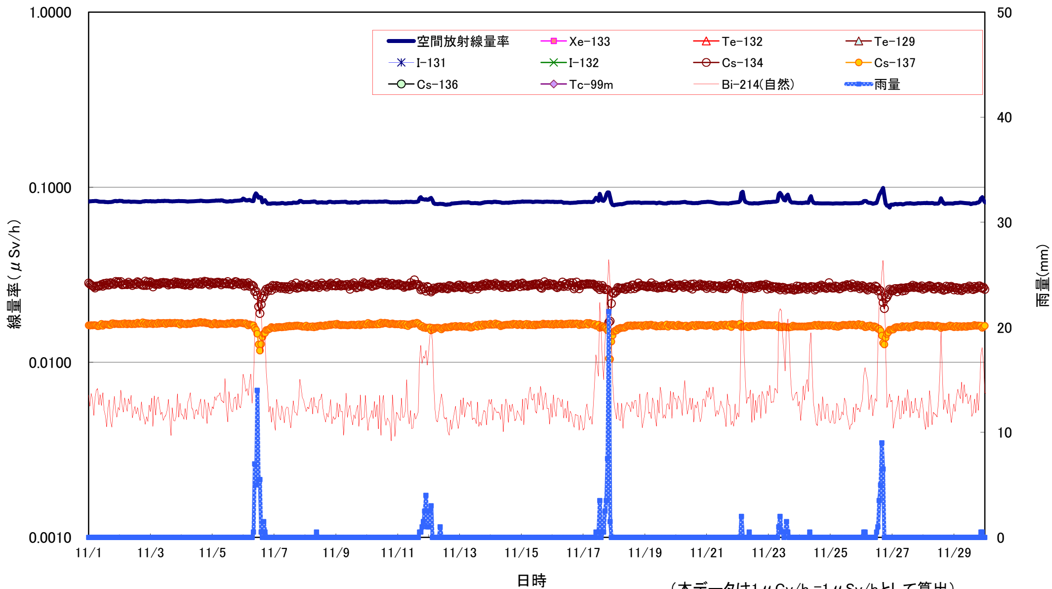
日本分析センターにおける空間放射線量率の測定結果(2012年11月)
