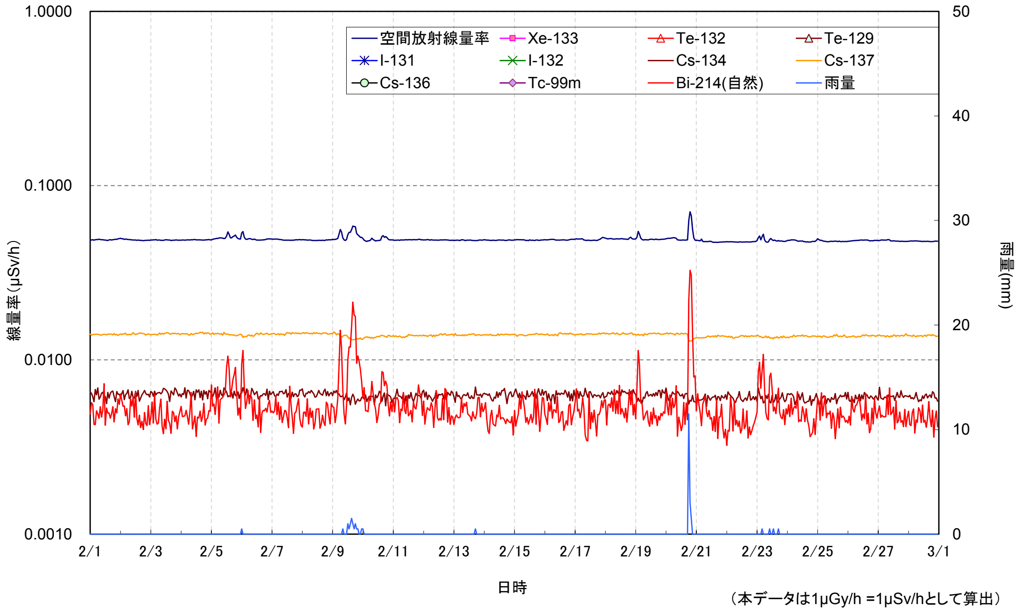
日本分析センターにおける空間放射線量率の測定結果(2017年2月)
