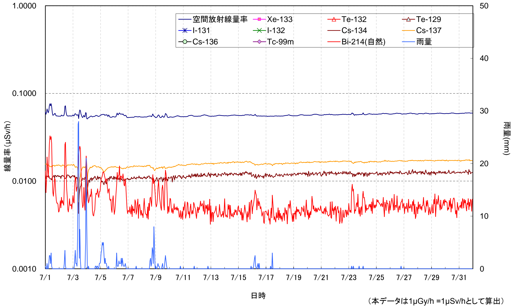
日本分析センターにおける空間放射線量率の測定結果(2015年7月)
